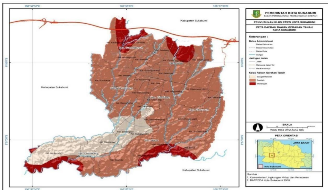
Gambar 2.5 Peta Rawan Gerakan Tanah di Kota Sukabumi
