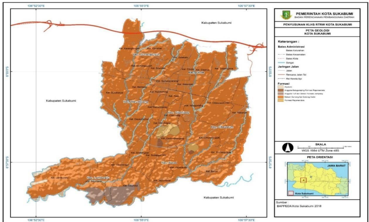
Gambar 2.6 Peta Geologi Kota Sukabumi
