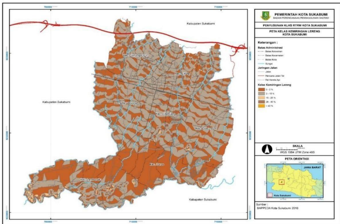
Gambar 2.4 Peta Kemiringan Lereng Kota Sukabumi
